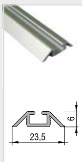
Spodné vedenie „W“ pre uchytenie v strede - Bott. guide rail „W“ for fixing in the middle - Alsó sín „W“ középen rögzítve - Dolný tor „W“ z mocowaniem w środku
