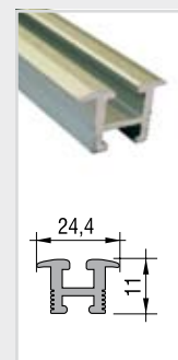
Spodné vedenie do dlažby - Bottom guide rail in paving - Bemart alsó sín - Dolný tor wpuszczany do glazury
