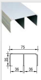
Vrchné vedenie - Upper guide rail - Felső sín - Görny tor UNIVERSAL
