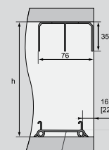
Spodné vedenie
