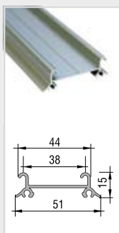
Spodné vedenie - Bottom guide rail - Alsó sín UNIVERSAL B
