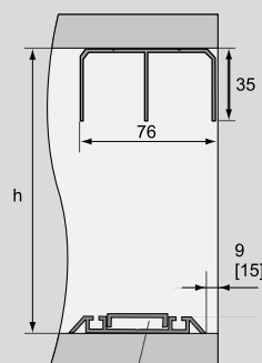
Spodné vedenie ELEGANT
