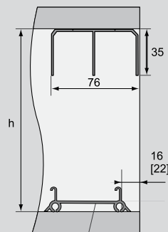
Spodné vedenie UNIVERSAL B
