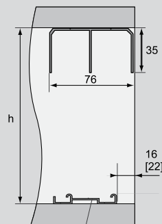
Spodné vedenie UNIVERSAL A
