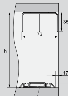
Spodné vedenie ELEGANT
