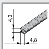
Dorazová nasúvacia bez lepidla
