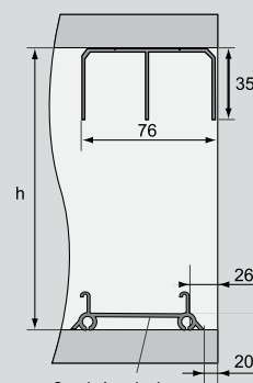
Spodné vedenie UNIVERSAL B
