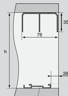
Spodné vedenie UNIVERSAL A
